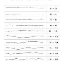
(그림 9) 거칠기 종단면과 JRC
